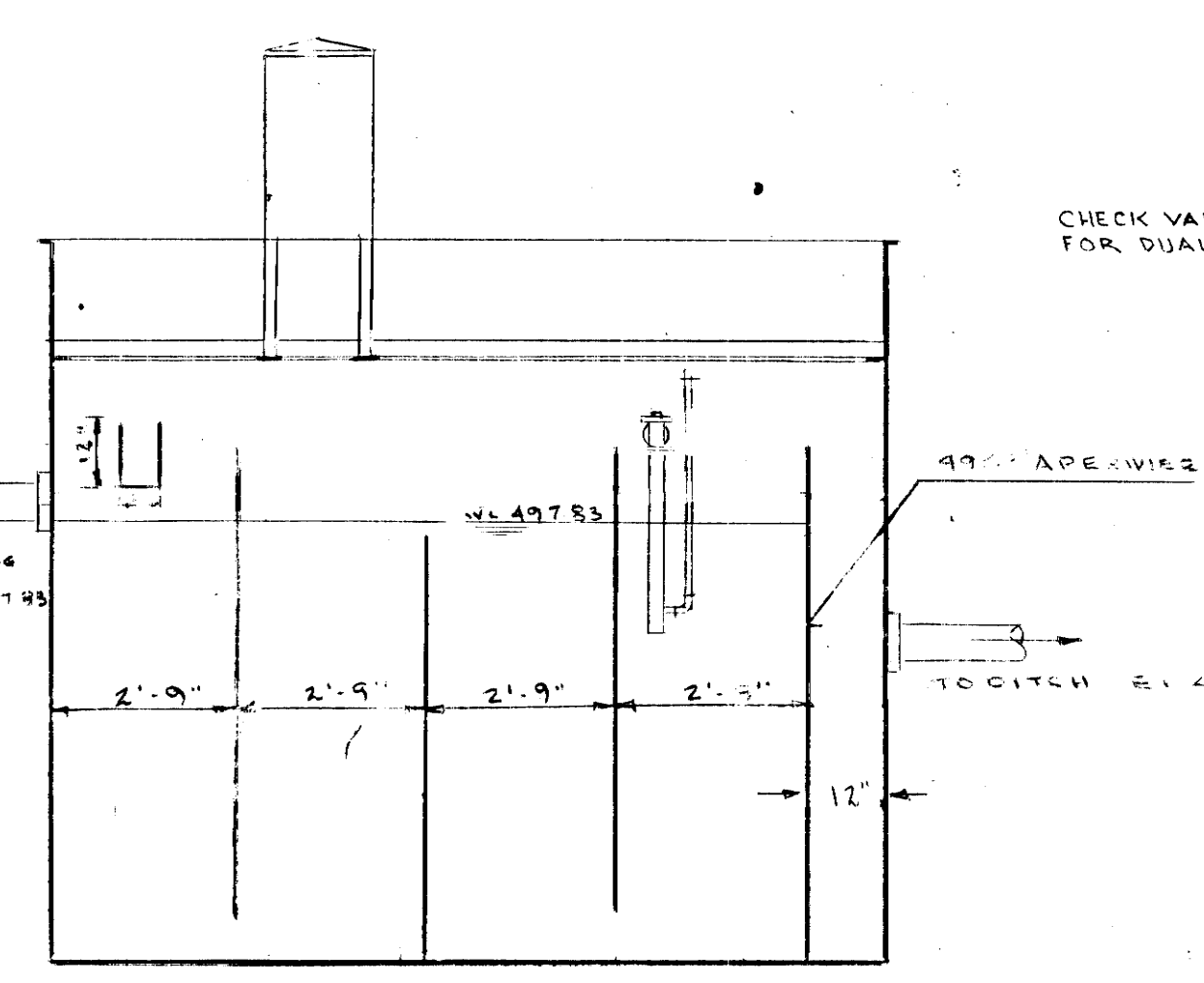
SECTION D-D
