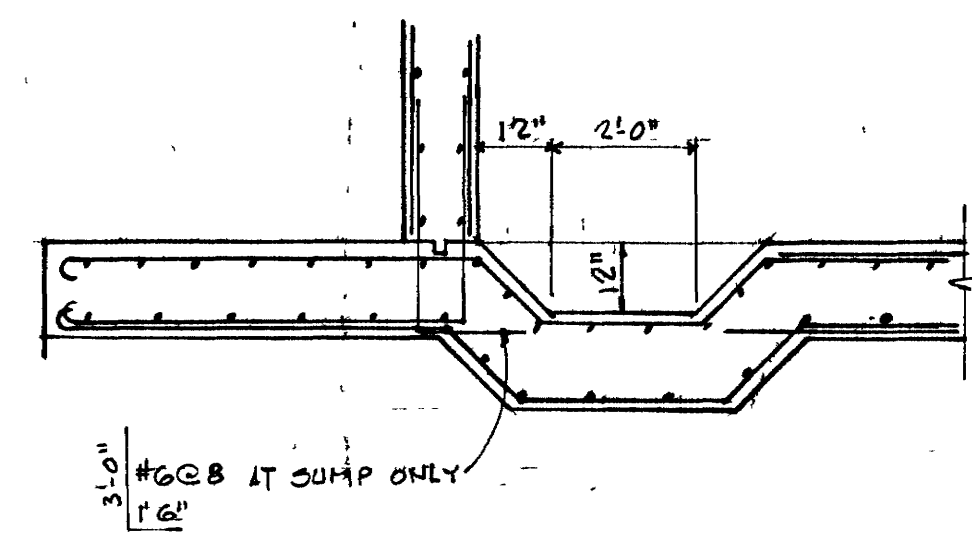
SECTION B SCALE: 3/8" = 1'-0"
