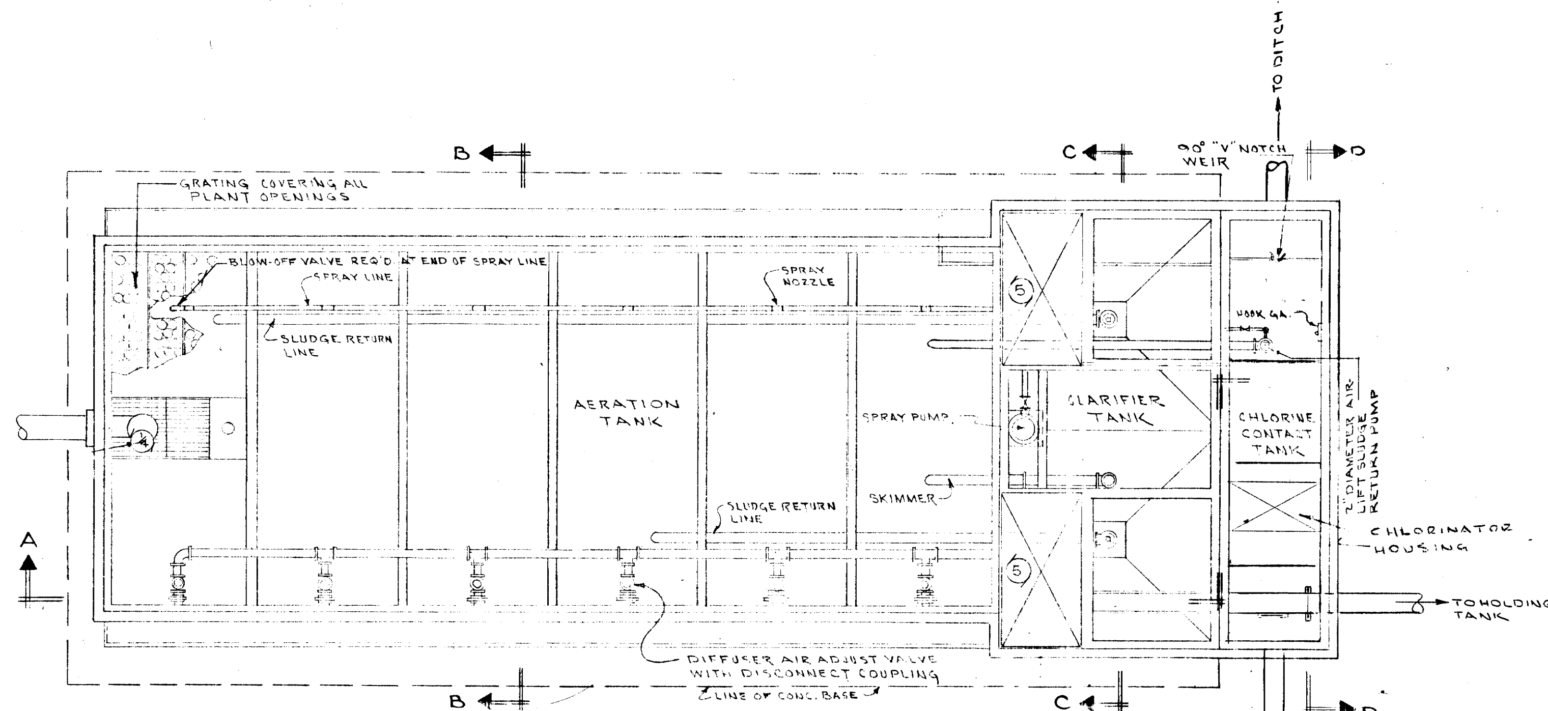
PLAN SCALE: 3/8"=1'-0"
