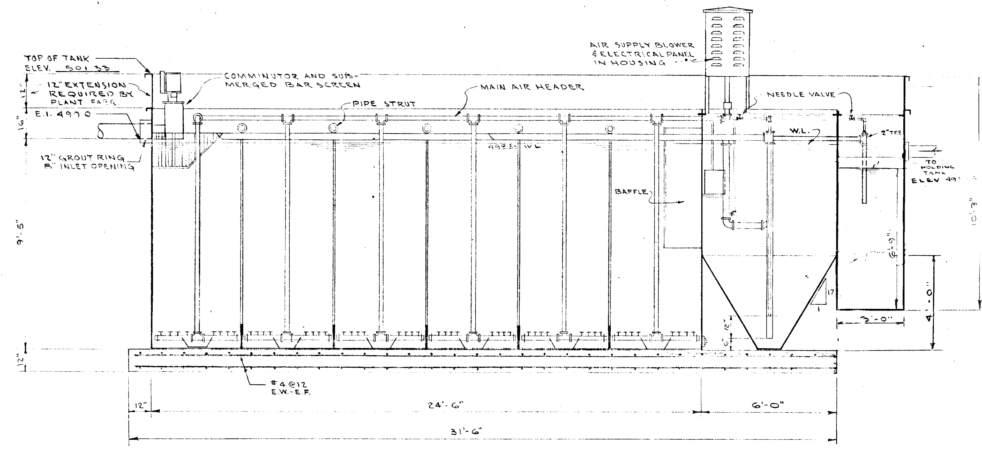
SECTION A-A
